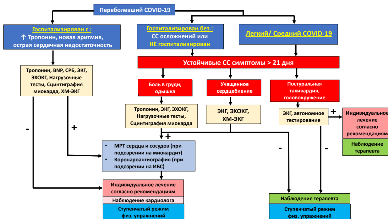
Рис. 4. Диагностический алгоритм
